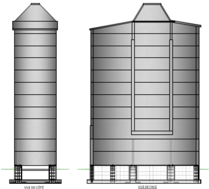
FONDATION SÉCHOIR À GRAIN
