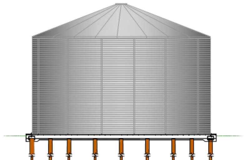
FONDATION SUR PIEUX POUR SILO
