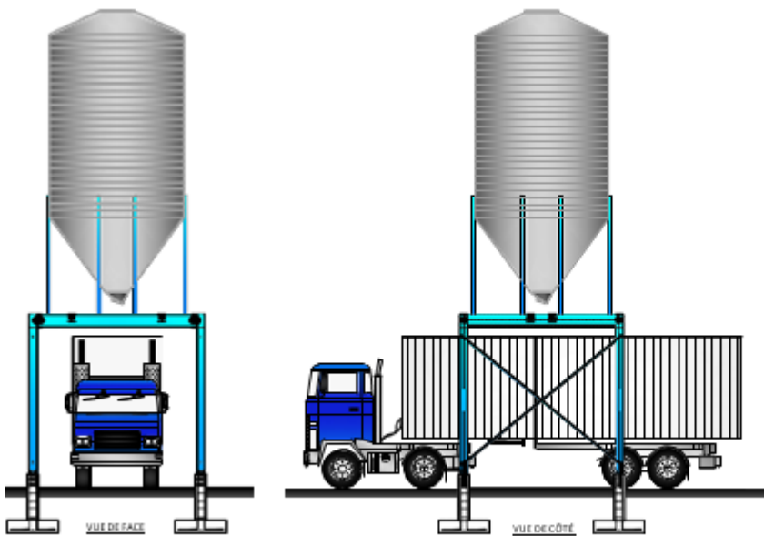
STRUCTURE D'ACIER ET FONDATION POUR SILO
